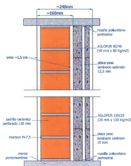
Figura 1 Sección vertical de la muestra ensayada
