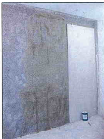
Imágenes 28, 29 y 30 PYL de 15 mm y su encolado sobre el panel AGLOPUR 150/20
