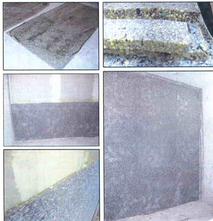
Imágenes 23, 24, 25, 26 y 27 Panel AGLOPUR 150/20 y su encolado sobre las PYL de 12,5 mm
