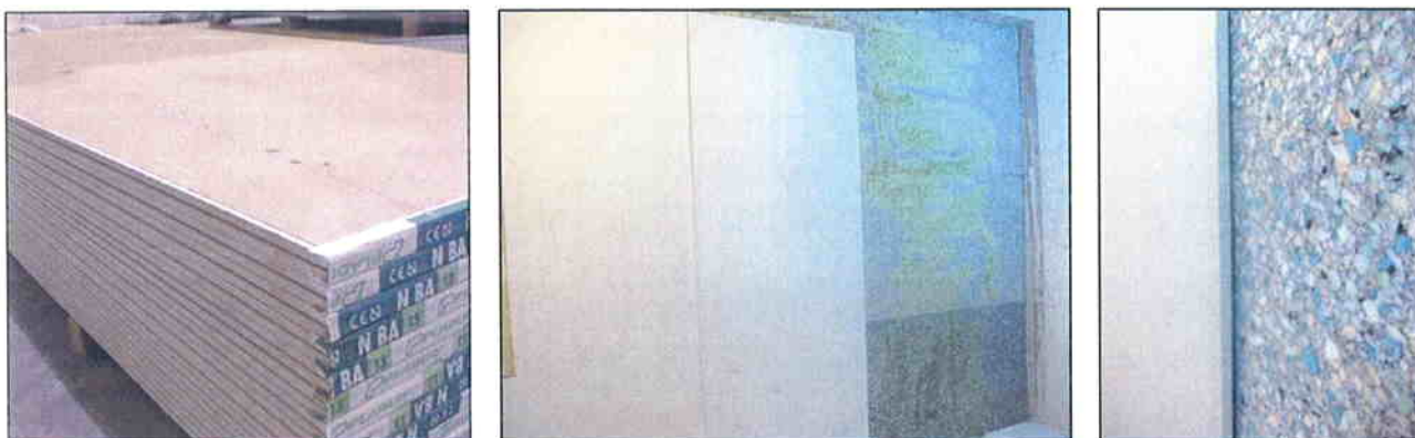
Imágenes 14, 15 y 16 PYL de 12,5 mm y su instalación sobre los paneles AGLOPUR
